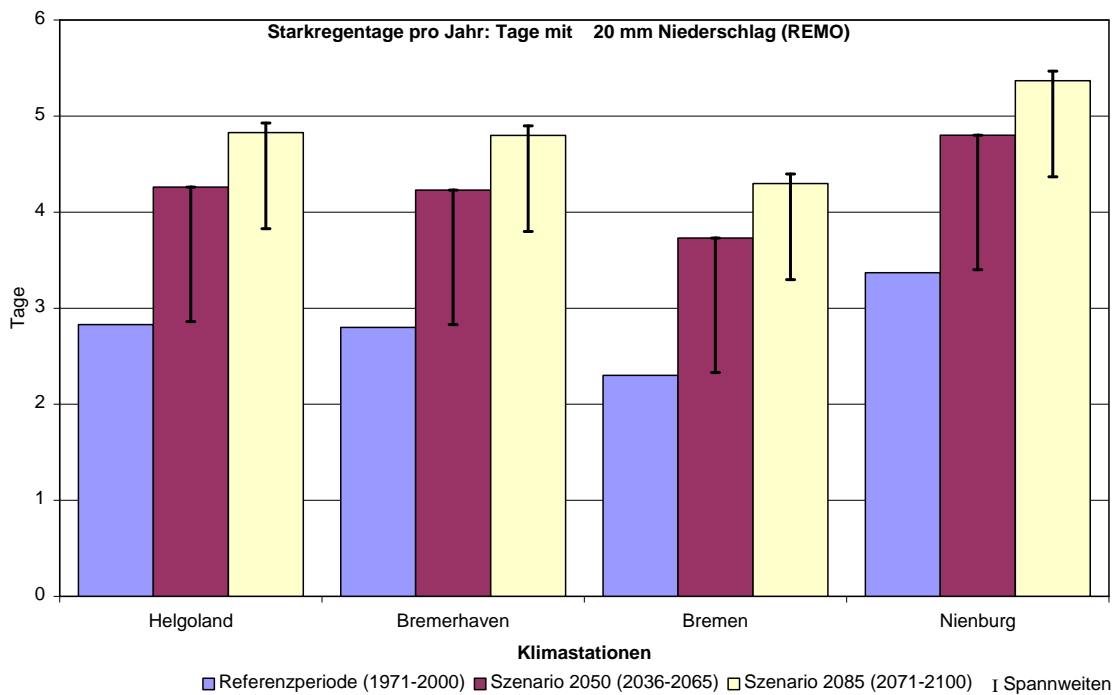
Abbildung 17: Mittlere Anzahl der Starkregentage pro Jahr für vier Klimastationen für die Referenzperiode sowie für die Szenarien 2050 und 2085 (oben CLM, unten REMO).
