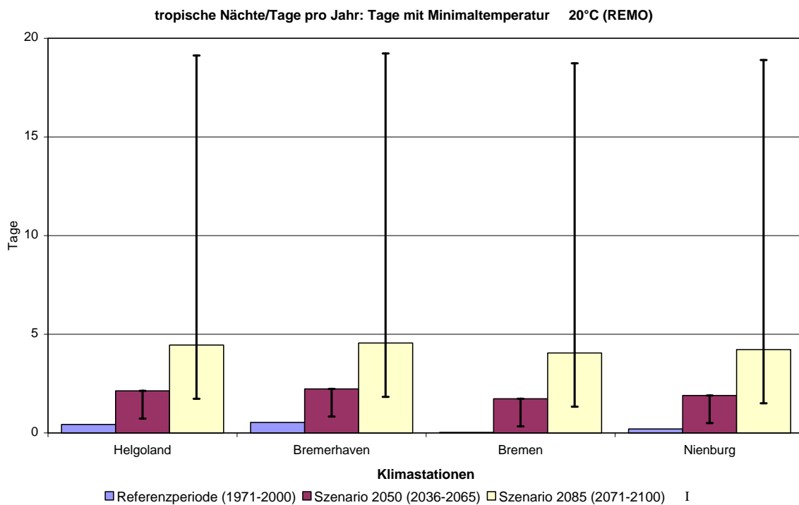
Abbildung 4: Mittlere Anzahl der tropischen Nächte pro Jahr für vier Klimastationen für die Referenzperiode sowie für die Szenarien 2050 und 2085 (oben CLM, unten REMO).
