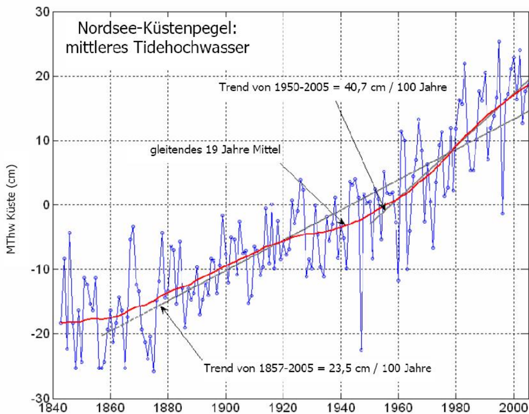
Abbildung 19: Normierte Zeitreihe für das MThw gemittelt für Nordsee-Küstenpegel (aus Jensen & Mudersbach 2007).
