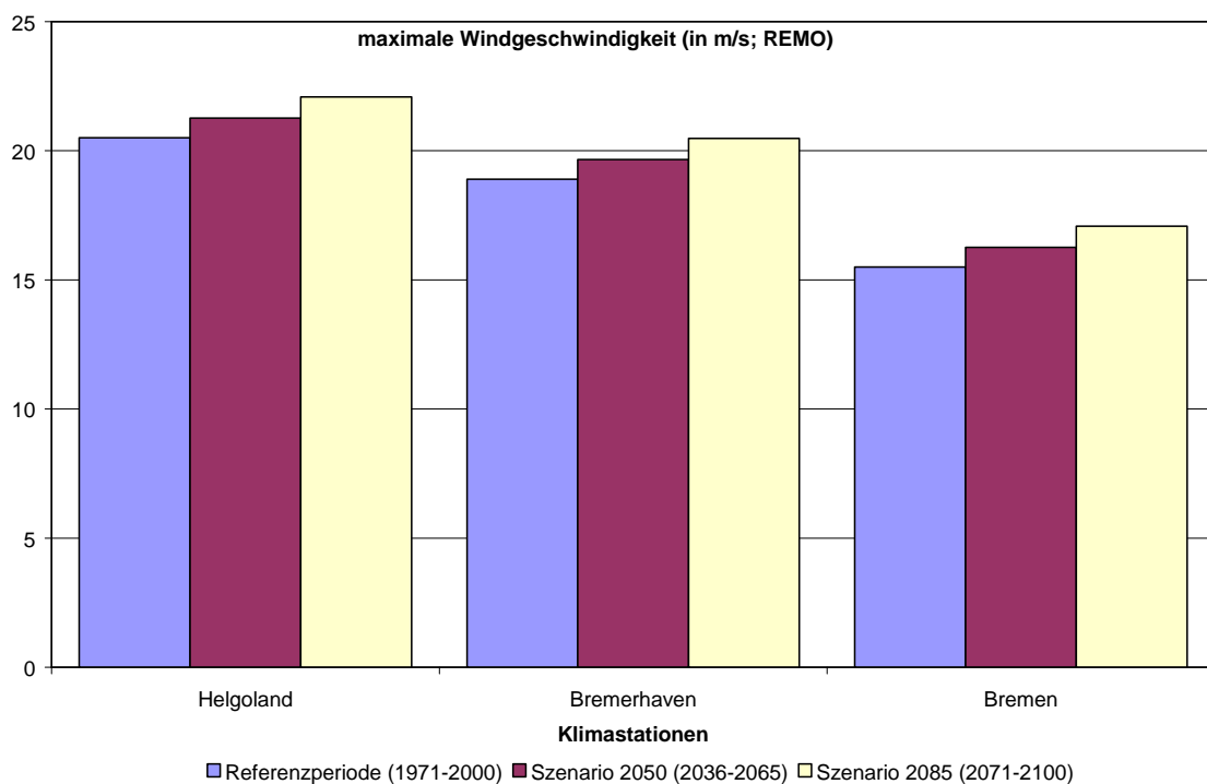
Abbildung 16: Maximale Windgeschwindigkeiten (Sturmintensitäten) für drei Klimastationen für die Referenzperiode sowie für die Szenarien 2050 und 2085 (oben CLM, unten REMO; Spannweiten sind nicht verfügbar).
