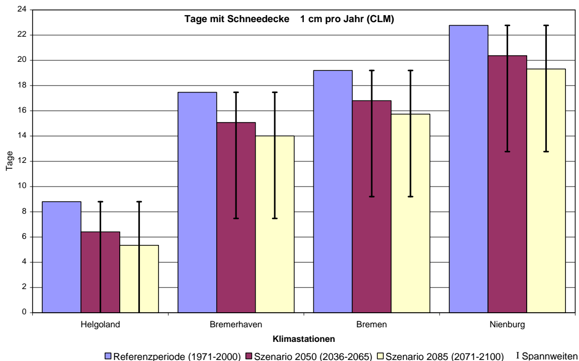
Abbildung 10: Mittlere Anzahl der Tage mit Schneedecke pro Jahr für vier Klimastationen für die Referenzperiode sowie für die Szenarien 2050 und 2085 (CLM).
