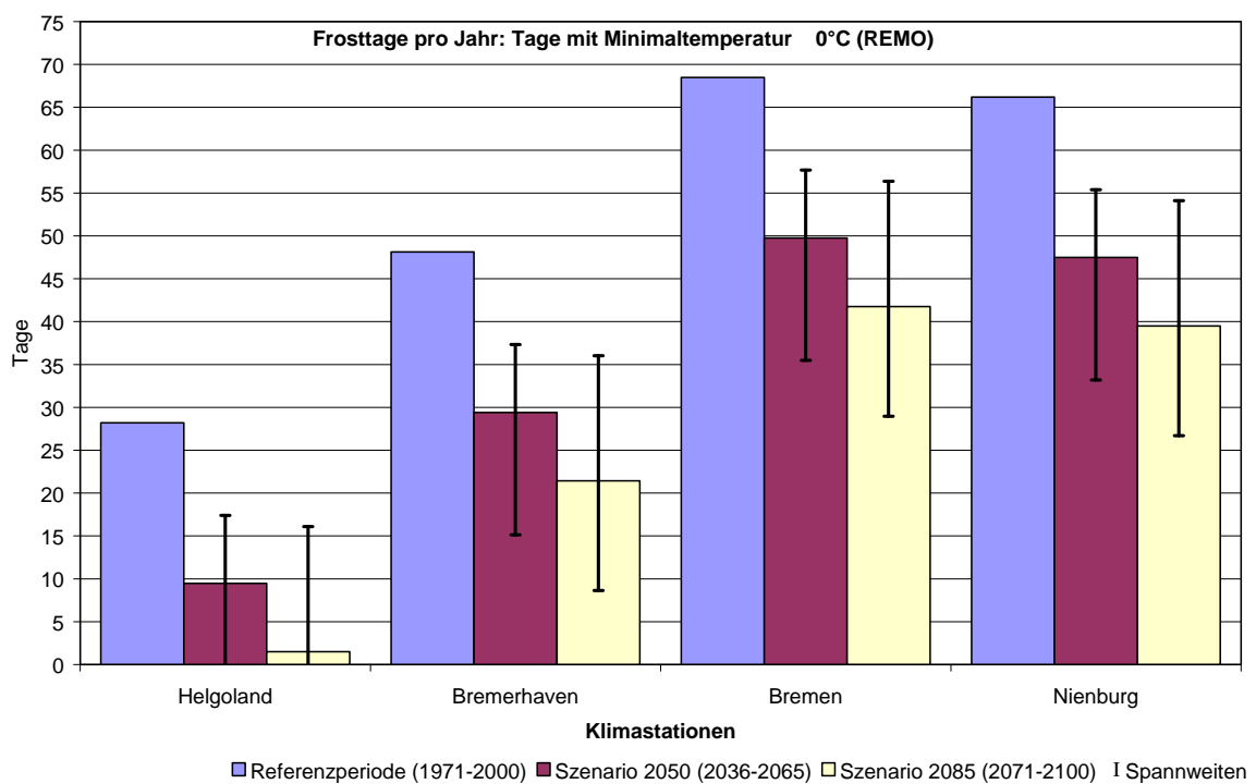
Abbildung 5: Mittlere Anzahl der Frosttage pro Jahr für vier Klimastationen für die Referenzperiode sowie für die Szenarien 2050 und 2085 (oben CLM, unten REMO).
