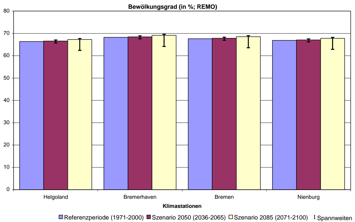
Abbildung 14: Mittlerer Bewölkungsgrad pro Jahr für vier Klimastationen für die Referenzperiode sowie für die Szenarien 2050 und 2085 (oben CLM, unten REMO).
