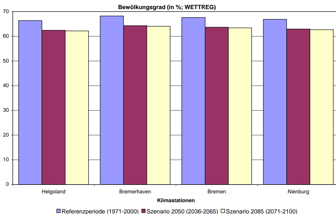
Abbildung 15: Mittlerer Bewölkungsgrad pro Jahr für vier Klimastationen für die Referenzperiode sowie für die Szenarien 2050 und 2085 (WETTREG).
