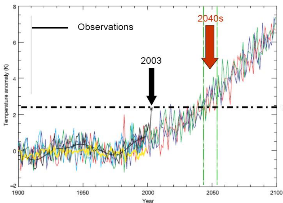
Abbildung 22: Temperaturanomalien der Monate Juni, Juli und August im Vergleich zur Periode 1961-1990 in Europa. Die gemessene Temperatur im Jahr 2003 ist als Sternchen dargestellt. Die schwarzen Linien stellen beobachtete bzw. gemittelte Temperaturen dar, die bunten Linien sind Modellierungsergebnisse des globalen Modells HadCM3 unter Berücksichtigung des A2 Szenarios (aus Lemke 2009).
