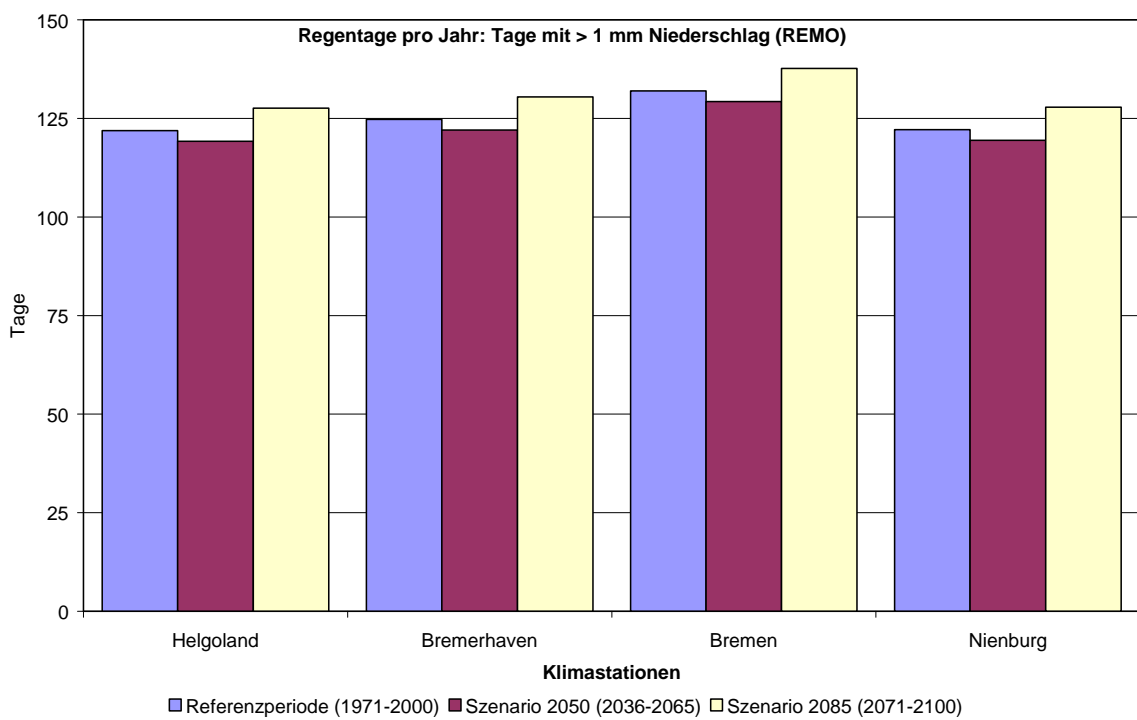
Abbildung 9: Mittlere Anzahl der Regentage pro Jahr für vier Klimastationen für die Referenzperiode sowie für die Szenarien 2050 und 2085 (oben CLM, unten REMO, Spannweiten nicht vorhanden).
