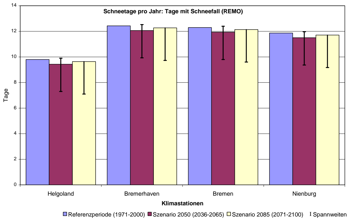
Abbildung 11: Mittlere Anzahl der Schneetage pro Jahr für vier Klimastationen für die Referenzperiode sowie für die Szenarien 2050 und 2085 (oben CLM, unten REMO).
