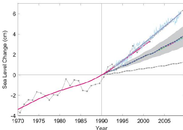
Abbildung 21: Veränderungen des mittleren globalen Meeresspiegels zwischen 1970 und 2008 im Vergleich mit 1990. Die durchgezogene dicke Linie basiert auf Messungen, die zur Entfernung interannueller Variabilität geglättet worden ist (Linie mit Datenpunkten) sowie die Projektionen des IPCC mit ihren Unsicherheitsbereichen (aus University of Copenhagen 2009).
