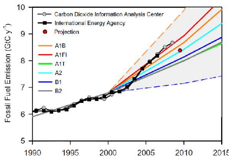
Abbildung 20: Angenommener Verlauf der CO 2 -Entwicklung nach IPCC-Emissionsszenarien und tatsächlicher Verlauf der Emissionen (nach GCP 2009; s.a. Raupach et al. 2007).
