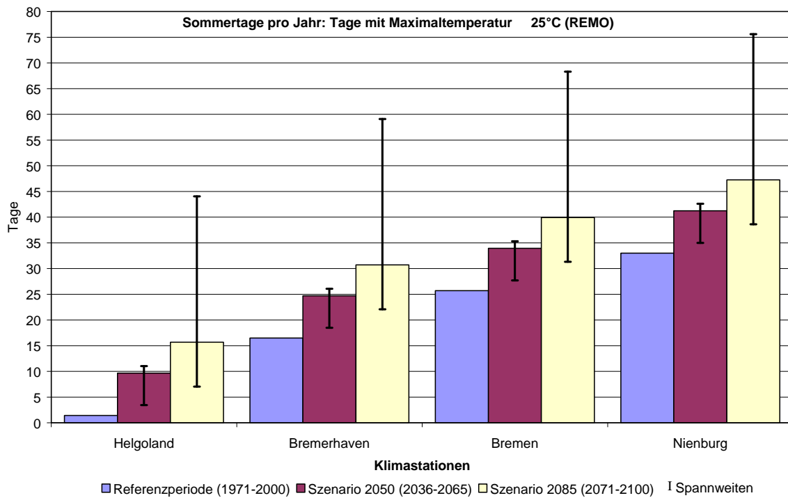
Abbildung 3: Mittlere Anzahl der Sommertage pro Jahr für vier Klimastationen für die Referenzperiode sowie für die Szenarien 2050 und 2085 (oben CLM, unten REMO).
