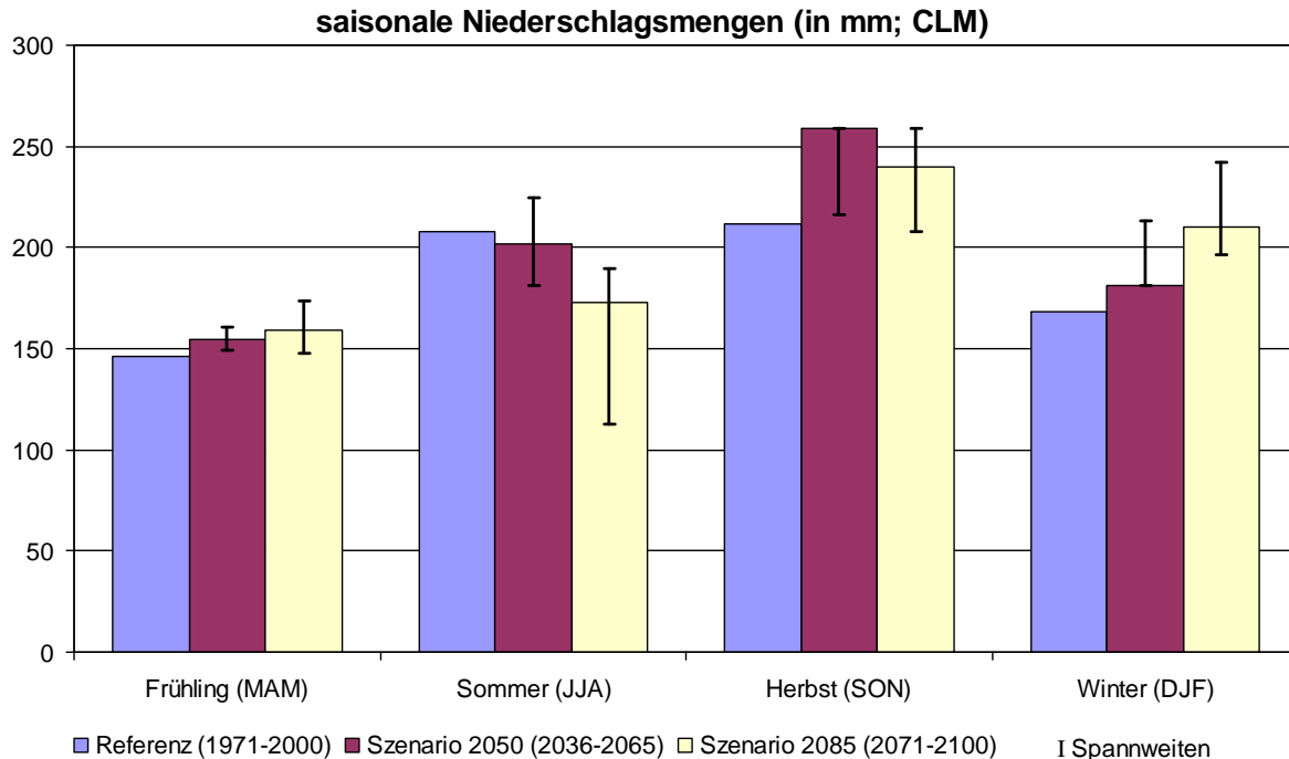
Abbildung 7: Saisonale Verteilung der Niederschlagsmengen für die Referenzperiode sowie die Szenarien 2050 und 2085 für CLM.
