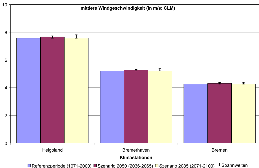
Abbildung 12: Mittlere jährliche Windgeschwindigkeit für drei Klimastationen für die Referenzperiode sowie für die Szenarien 2050 und 2085 (CLM).
