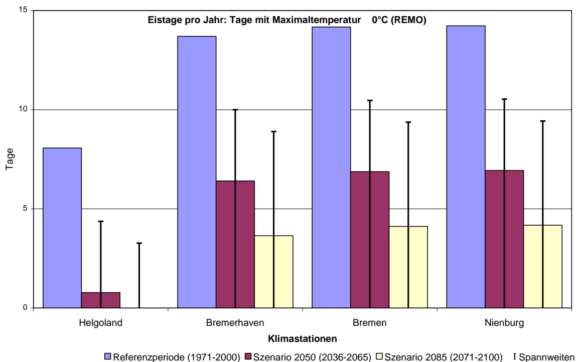
Abbildung 6: Mittlere Anzahl der Eistage pro Jahr für vier Klimastationen für die Referenzperiode sowie für die Szenarien 2050 und 2085 (oben CLM, unten REMO).
