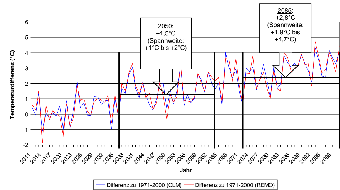
Abbildung 2: Temperaturdifferenzen der durchschnittlichen Jahresmittel aus den Regionalmodellen CLM und REMO im Vergleich mit der Referenzperiode 1971-2000.
