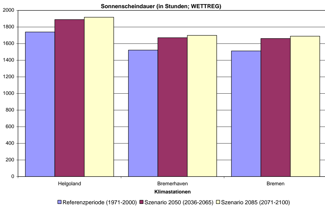
Abbildung 13: Mittlere jährliche Sonnenscheindauer für drei Klimastationen für die Referenzperiode sowie für die Szenarien 2050 und 2085 (CLM oben, WETTREG unten und ohne Spannweiten).
