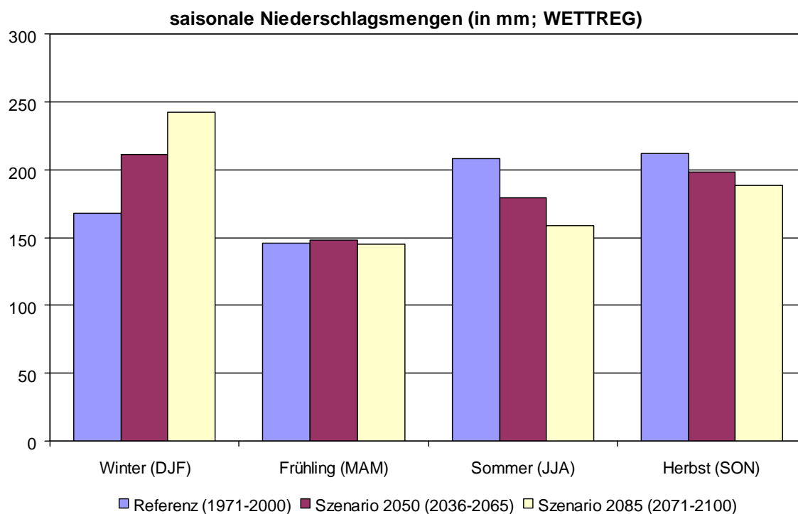
Abbildung 8: Saisonale Verteilung der Niederschlagsmengen für die Referenzperiode sowie die Szenarien 2050 und 2085 für WETTREG (keine Spannweitenbetrachtung).
