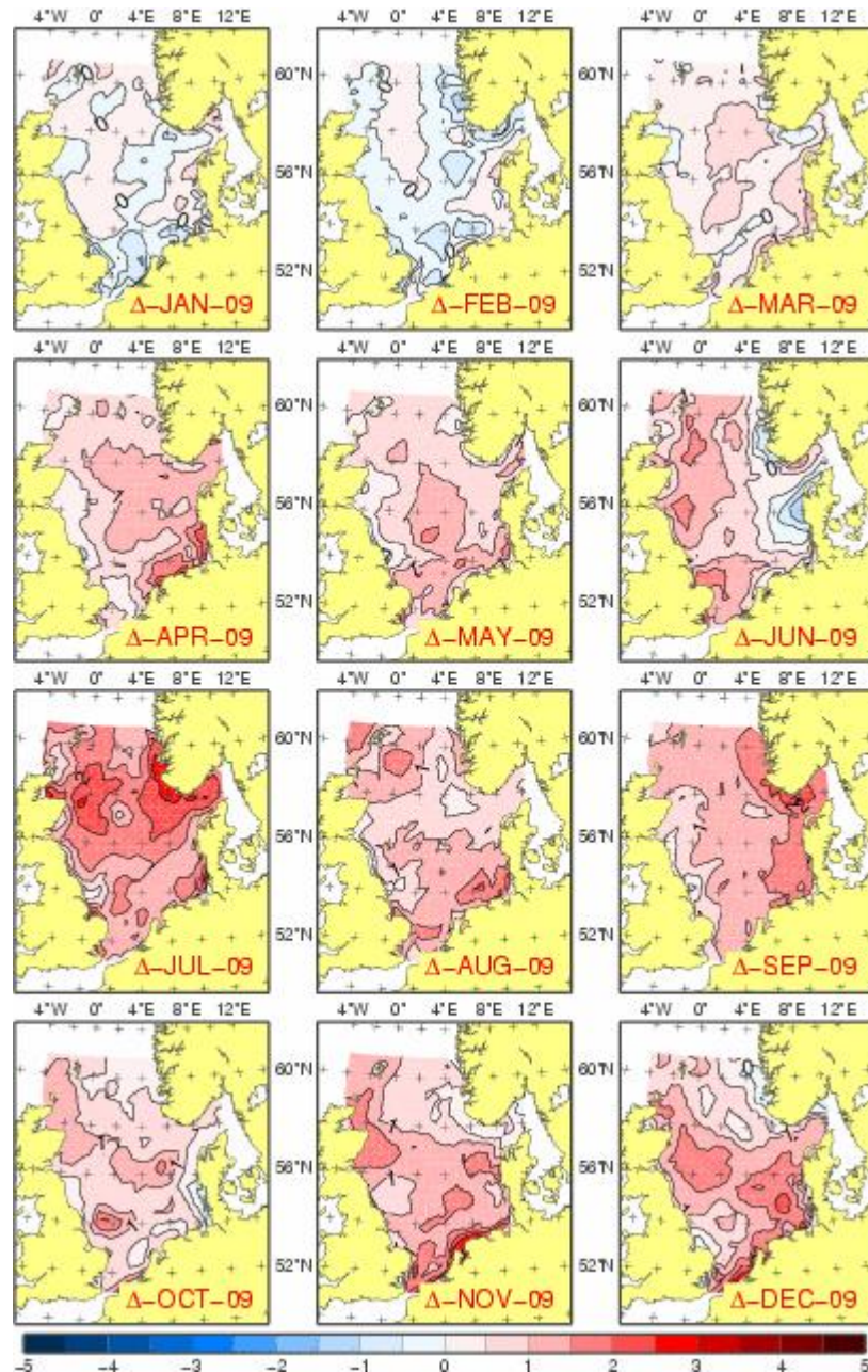
Abbildung 18: Temperaturanomalien in den Wassertemperaturen der Nordsee für das Jahr 2009. Die Anomalien der raumzeitlichen Temperaturfelder sind vom BSH aus den wöchentlichen Oberflächentemperaturfeldern für den Zeitraum 1971-1993 anhand einer monatlichen Klimatologie berechnet worden ( http://www.bsh.de/ ).
