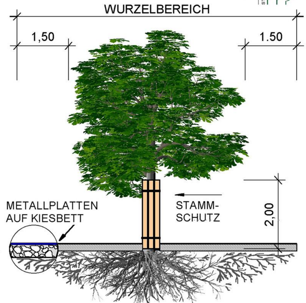
WURZELSCHUTZ DURCH LASTVERTEILUNG
