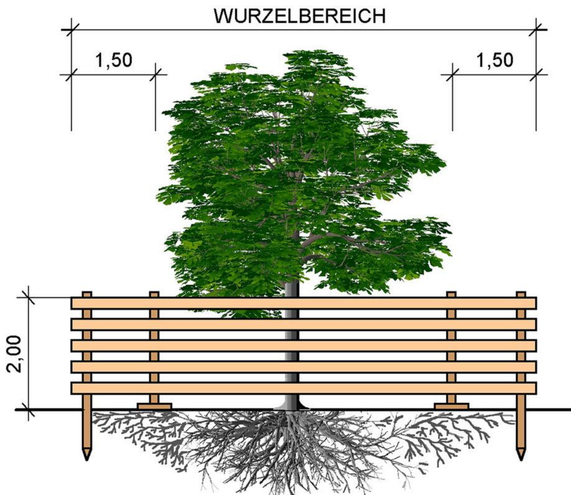
WURZELSCHUTZ DURCH ZAUN
